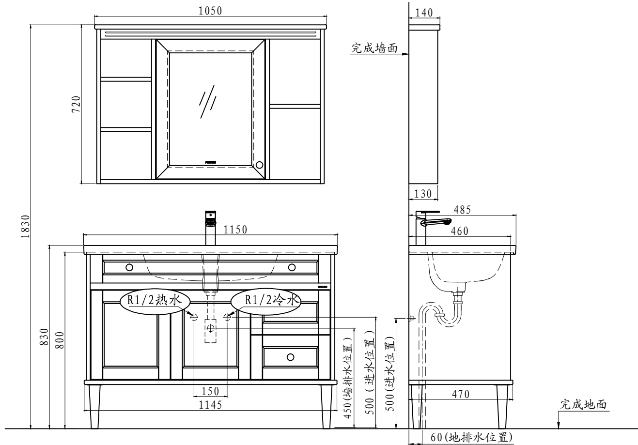
FPGM3688J 实木柜水电安装图 (建议安装尺寸)
